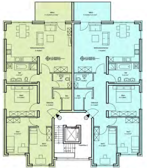
Wohnung 3.3 Haus 3 Wohnung 3.4
