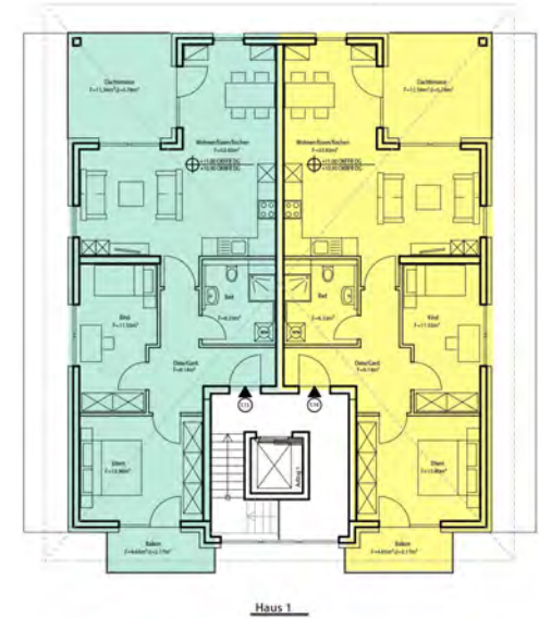
Wohnung 1.13 Wohnung 1.14
